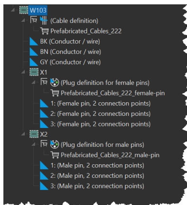
Abbildung 5: Nicht-platziertes vorkonfektioniertes Kabel mit Artikeln im Betriebsmittel-Navigator.
