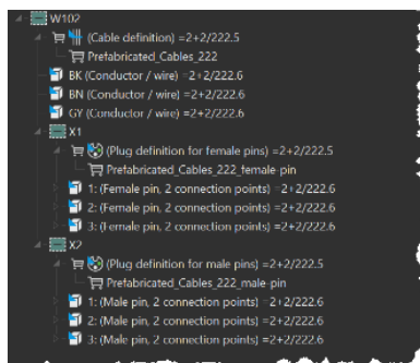
Abbildung 6: Platziertes vorkonfektioniertes Kabel mit Artikeln im Betriebsmittel-Navigator.
